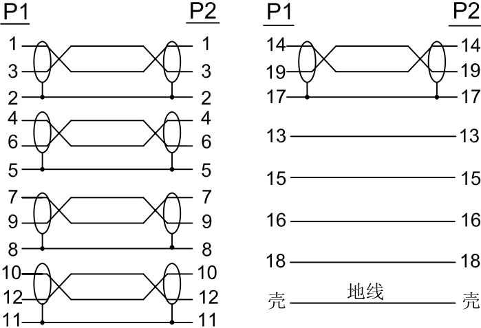
接线图
